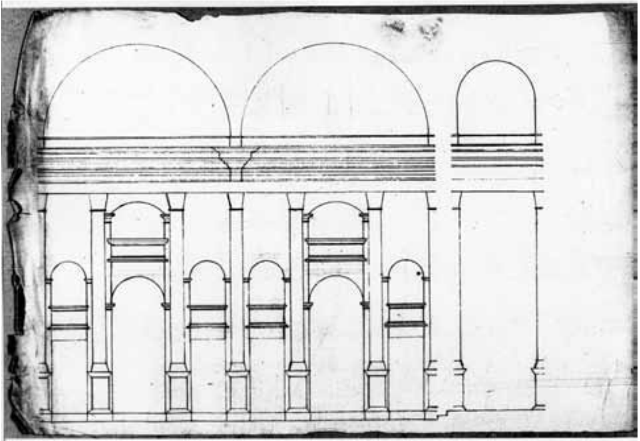
60. Como, Plan Nr. 3, Längsschnitt.
