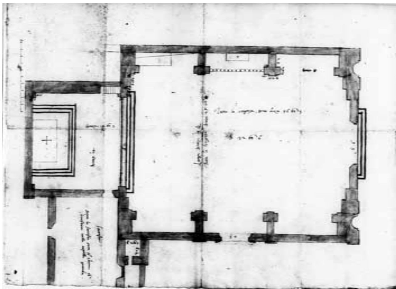
58. Como, Plan Nr. 1.
