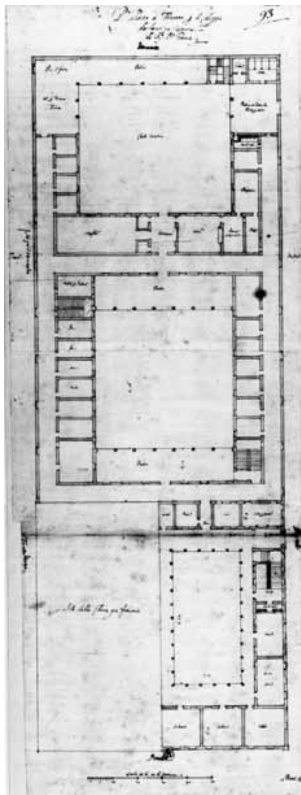
72. Cremona, Plan Nr. 4.
